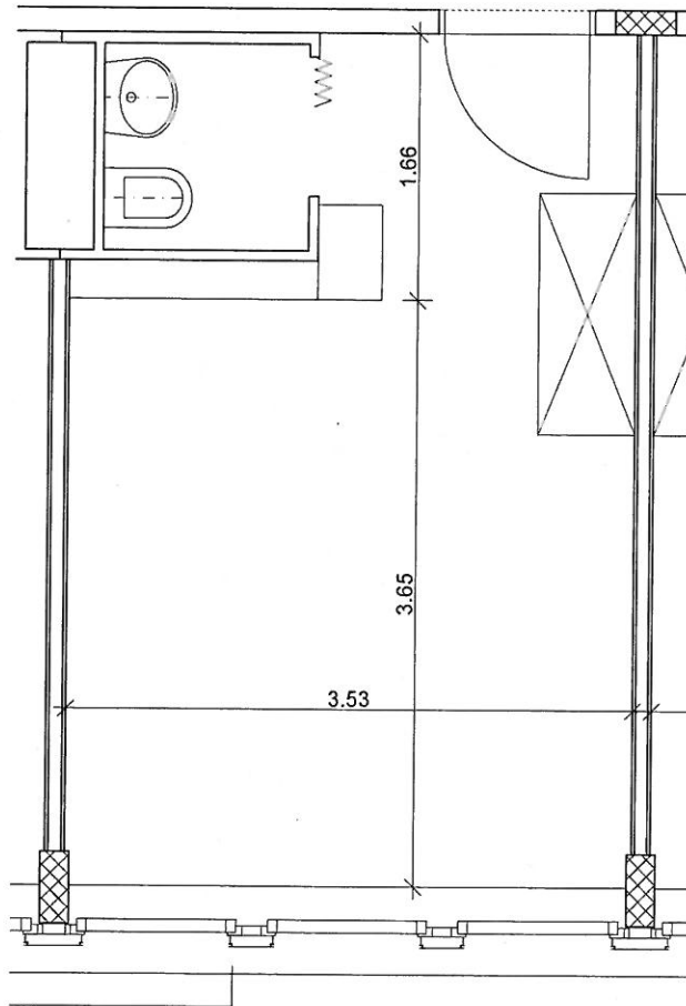
Übersicht Zimmer 306, 1:50 ohne Möbel
